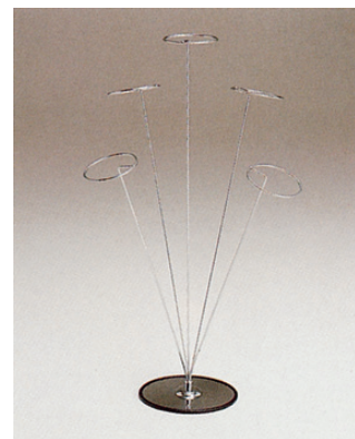
4 K1423-5 帽子掛け W.250 × D.195 × H.730 ベース：φ 195 厚み7
