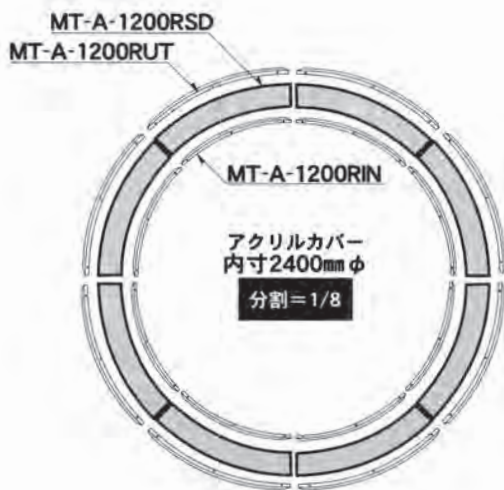
サークルトラス2400用アクリルカバー
