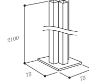
RAL-6 (T型アーム)
