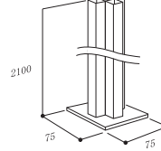
RAL-7 (十字型アーム)
