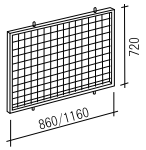
NS-15 ネットパネル上部フレーム用1200タイプ NS-15-900 ネットパネル上部フレーム用 900タイプ
