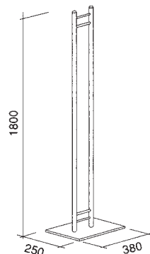
柱 B H1800 SR-2
