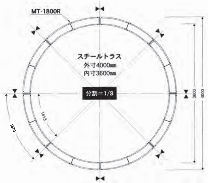
スチールサークルトラス3600
