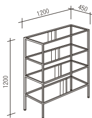
NS-19 4段ガラス棚
