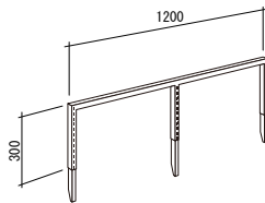
UFM-6W バックフレーム H300 継足しパーツ (白) UFM-6B バックフレーム H300 継足しパーツ (黒)
