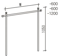
NS-5-600 -900 -1200 丸パイプシングルハンガー
