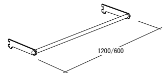
RP-55 ハンガーバーセット1200タイプ RP-55-600 ハンガーバーセット 600タイプ
