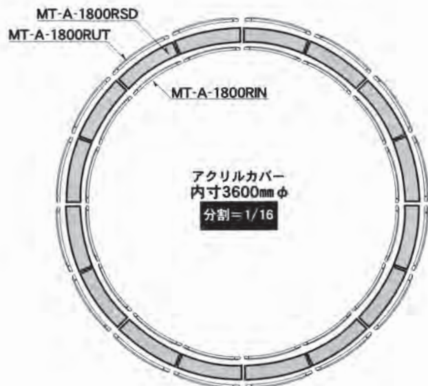
サークルトラス3600用アクリルカバー
