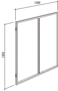
UFM-2W バックフレーム H1350 (白) UFM-2B バックフレーム H1350 (黒)
