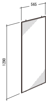
UFM-10W バックパネル H1350 (白) UFM-10B バックパネル H1350 (黒) UFM-10SN バックパネル H1350 (シナ合板)
