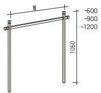
NS-6-600 -900 -1200 角パイプシングルハンガー
