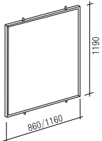
NS-16W パネル本体用 白1200タイプ NS-16B パネル本体用 黒1200タイプ NS-16K パネル本体用 こげ茶1200タイプ NS-16N パネル本体用 格子1200タイプ NS-16W-900 パネル本体用 白1200タイプ NS-16B-900 パネル本体用 黒1200タイプ NS-16K-900 パネル本体用 こげ茶1200タイプ NS-16N-900 パネル本体用 格子1200タイプ
