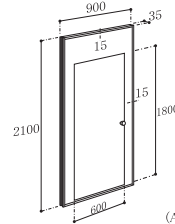
[アルファドア付パネル]
